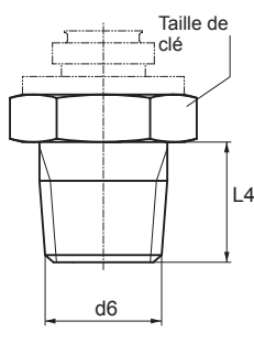
Filetages coniques
