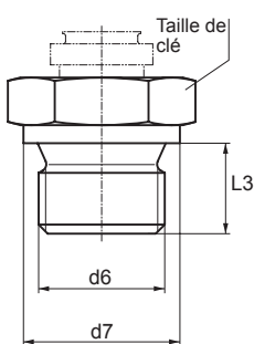
Filetages cylindriques
