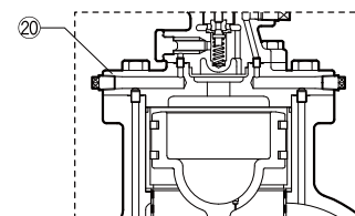
Couvercle
